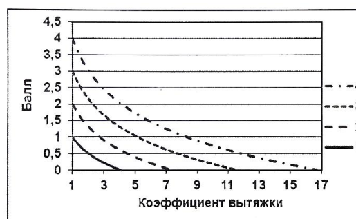
Рис. 2. Вплив коефіцієнта витяжки на проробку макроструктури безперервнолитої заготовки: 1, 2, 3, 4 – бал центральної (осьової) пористості та ліквіації в макроструктурі БЛЗ [26]
