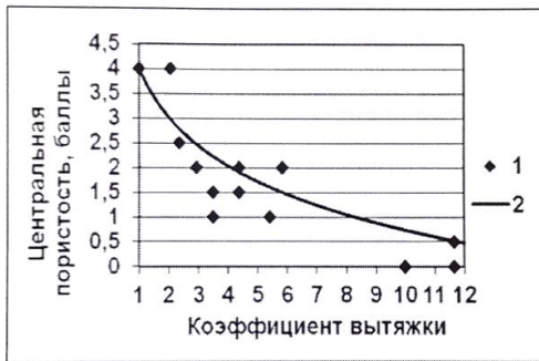
Рис. 3. Порівняння розрахункових даних з експериментальними даними [26]: 1 – експериментальні дані [28]; 2 – розрахункові дані
