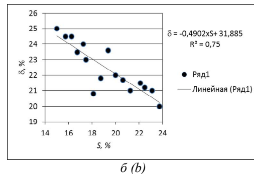
Рис. 2. Співвідношення між механічними властивостями та вмістом перліту в сталі 15пс / Fig. 2. The ratio between the mechanical properties and the content of perlite in steel 15пс
